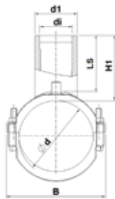
180-63 מ"מ עם יציאות 32 עד 63 מ"מ
